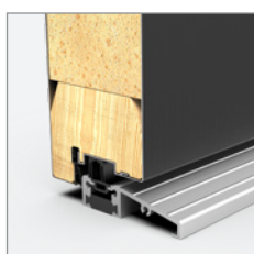
4 przylgi skrzydła
